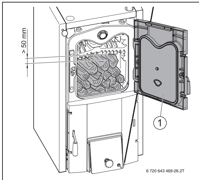
Рис. 9 Дозагрузка дров
